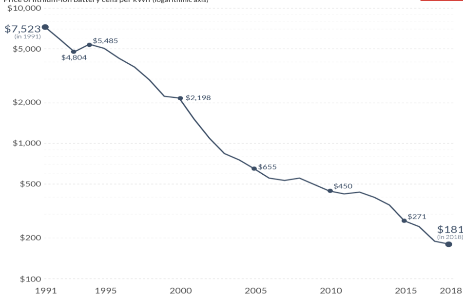
Figura 4- Redução do custo de baterias desde 1991 The price of lithium-ion batteries fell by 97%
