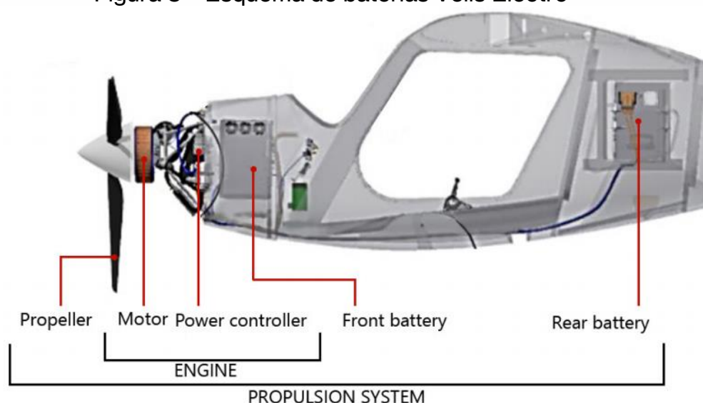
Figura 3 – Esquema de baterias Velis Electro
