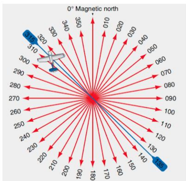
Figura 7 - Funcionamento do VOR
