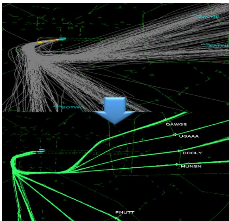
Figura 21 - Comparativo 1 de tráfego em navegação convencional e RNAV
