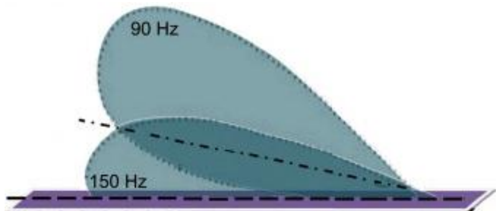
Figura 10 - Trajetória do Glide Slope
