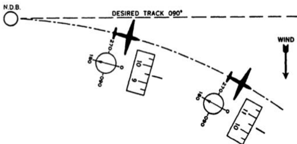
Figura 5 - Funcionamento do NDB
