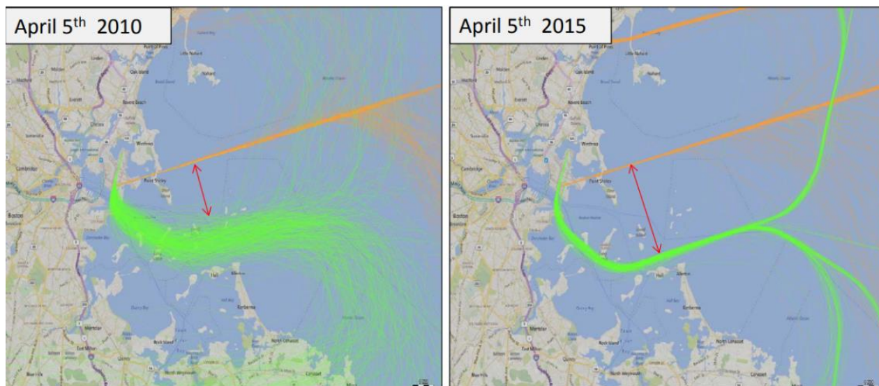
Figura 23 - Distância segura entre aproximação e perfil de saída
