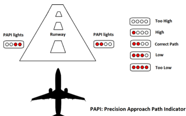
Figura 17 - PAPI
