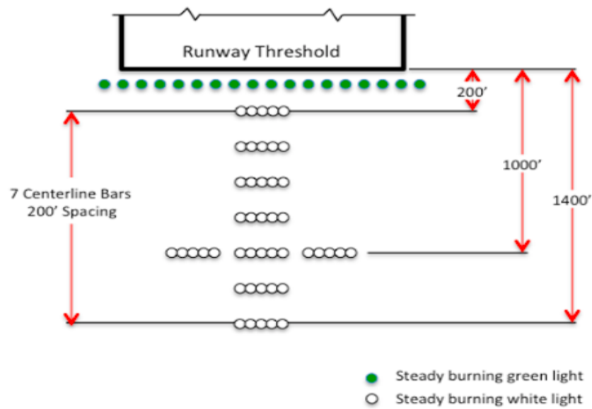
Figura 14 - MALS
