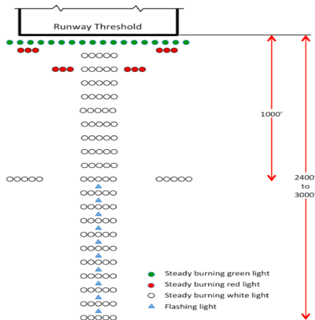
Figura 13 - ALSF-1
