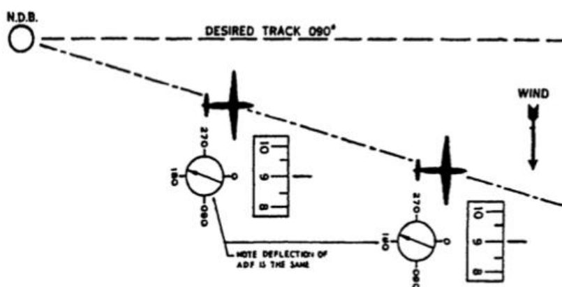
Figura 6 - Efeito do vento no uso do NDB
