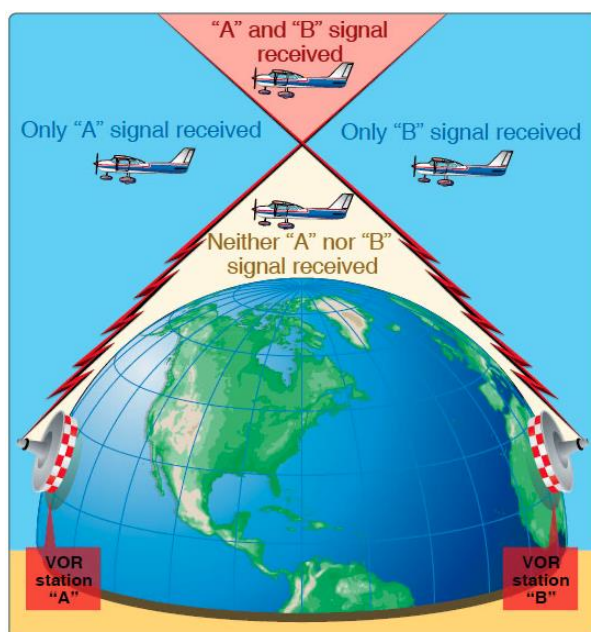
Figura 8 - Alcance de recepção do VOR
