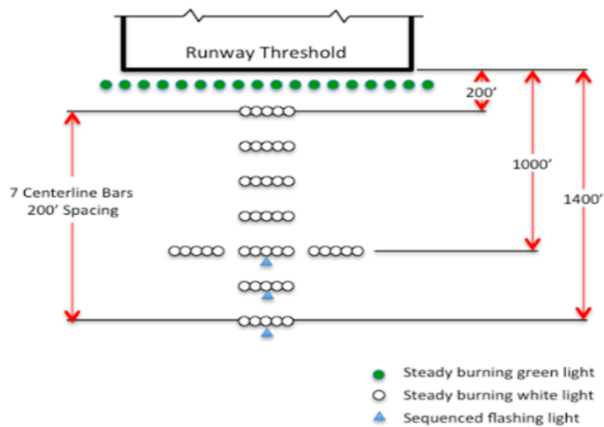
Figura 15 - MALSF
